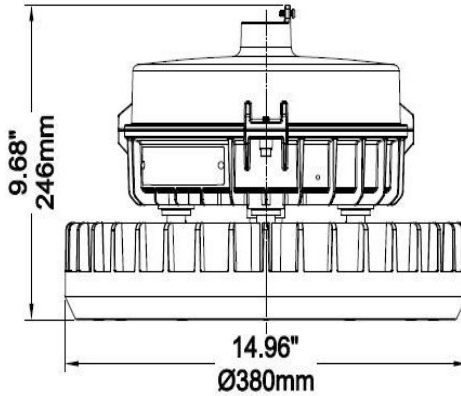
Pendant mount
